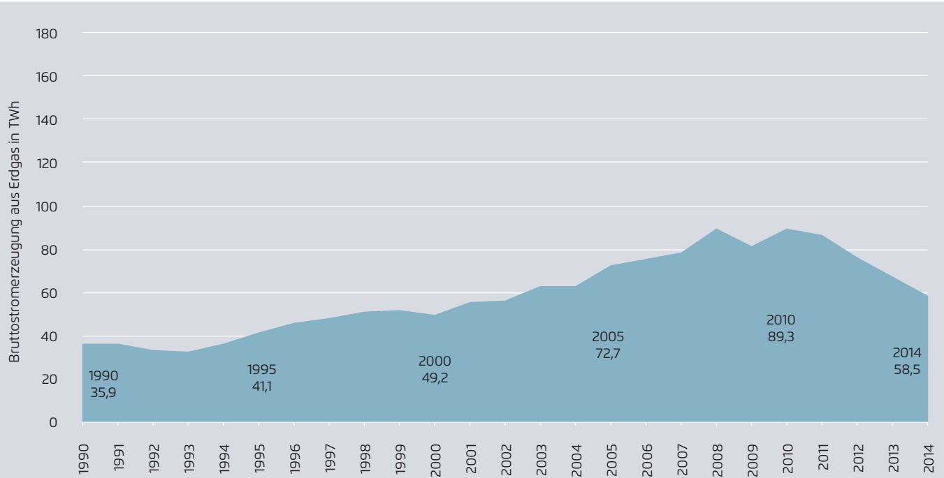
Die Stromerzeugung aus Erdgas erfolgte 2014 fast nur noch in KWK-Anlagen.
